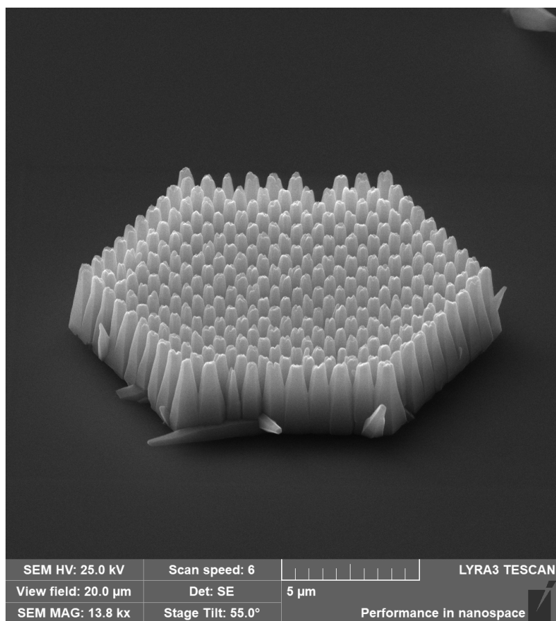
Figure 3: Snímek úspěšně připraveného uspořádaného pole nanotyček s rozstupem 0,8 \mu\text{m} narostlého v reaktoru s kontinuálním průtokem. Pořízeno rastrovacím elektronovým mikroskopem. Pohled z náklonu 55^\circ oproti rovině substrátu.
