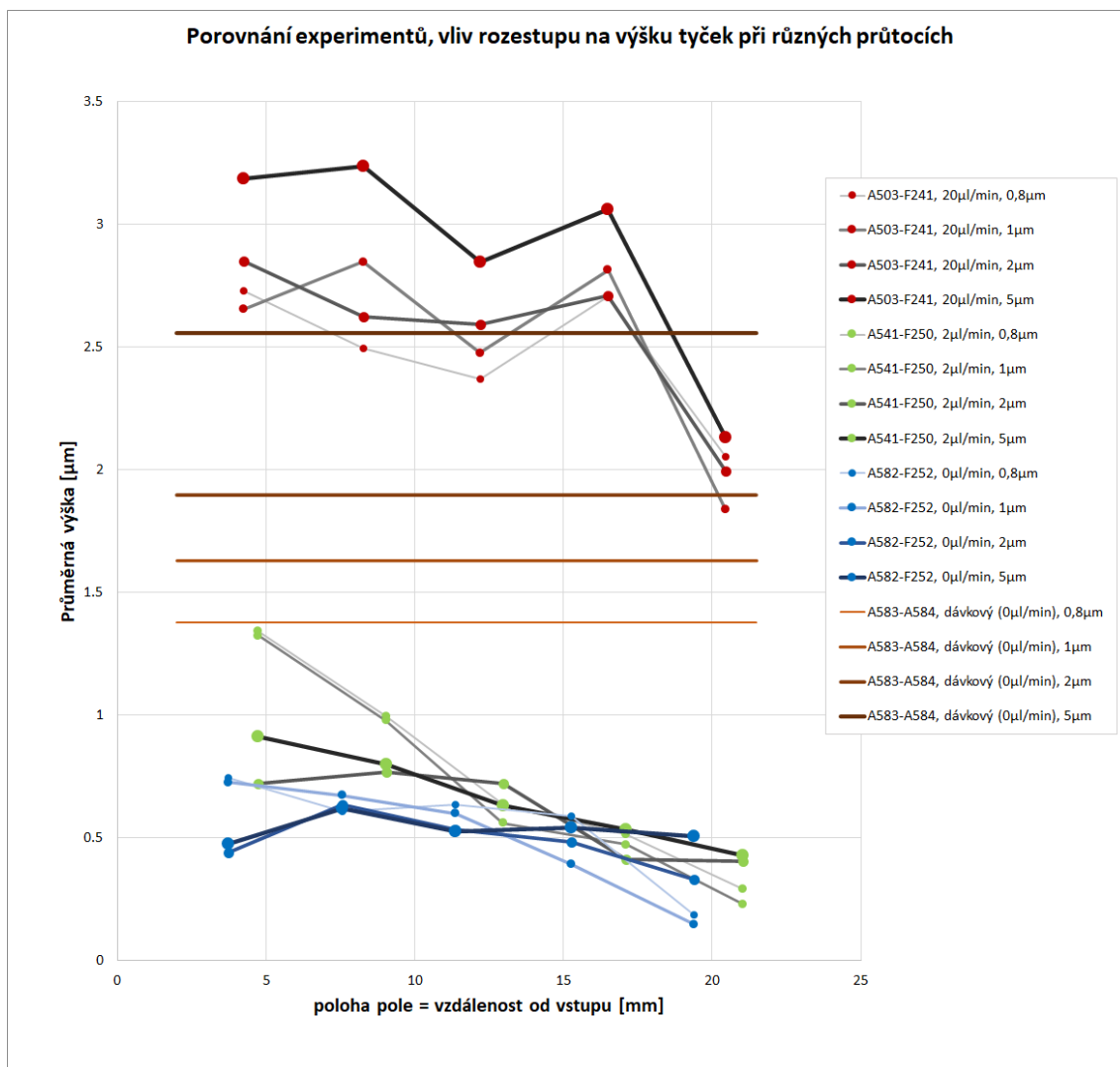
Figure 4: Graf závislosti vlivu rozestupu mezi nanotyčkami, rychlosti průtoku roztoku průtokovým reaktorem a vzdálenosti od vstupu do reaktoru na průměrnou výšku nanotyček na uspořádaném poli. Hodnoty rychlosti průtoku: 20, 2, 0 μl/ min a srovnání s průměrnými výškami v dávkovém reaktoru (hnědé úsečky); hodnoty rozestupů: 0,8; 1; 2; 5 μm.
