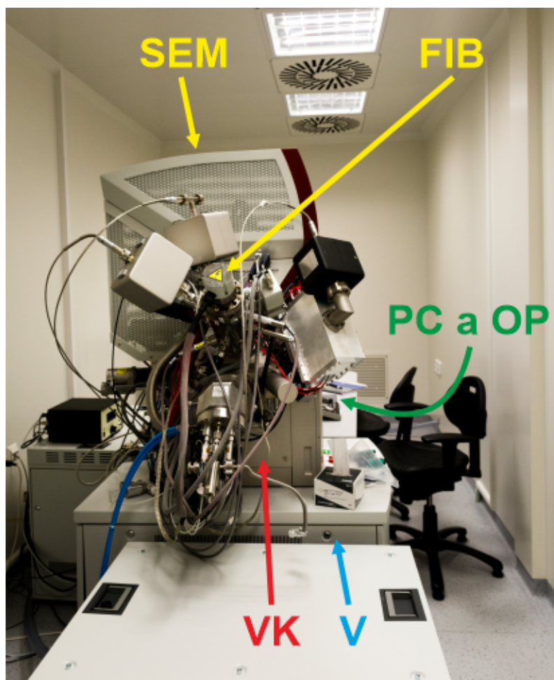
Figure 2: Pohled na víceúčelový mikroskop Tescan LYRA 3. SEM – Scanning Electron Microscope (Rastrovací (skenovací) elektronový mikroskop), FIB – Focused Ion Beam Microscope (Mikroskop využívající fokusovaný iontový svazek), PC a OP – počítač a ovládací prvky, VK – vakuová komora, V – vývěvy. Obrázek z archivu ÚFE, upraveno.
